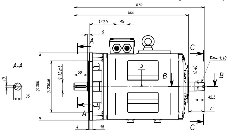
Габаритный чертеж Dimension drawing
